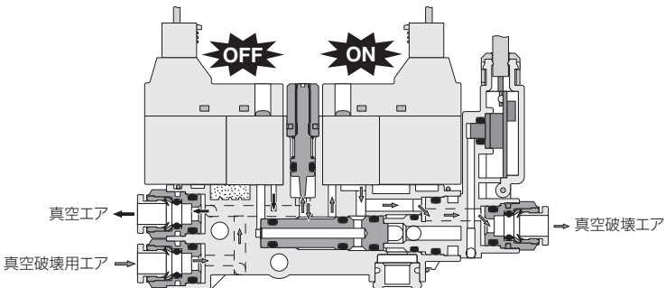
③.真空破壊用電磁弁ON時(真空破壊エア供給)
