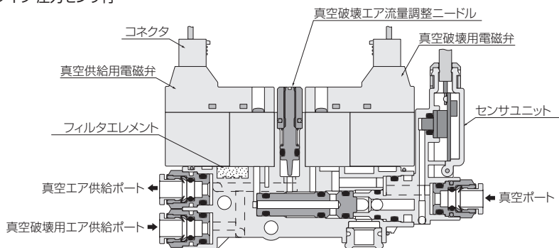
単体タイプ 圧力センサ付
