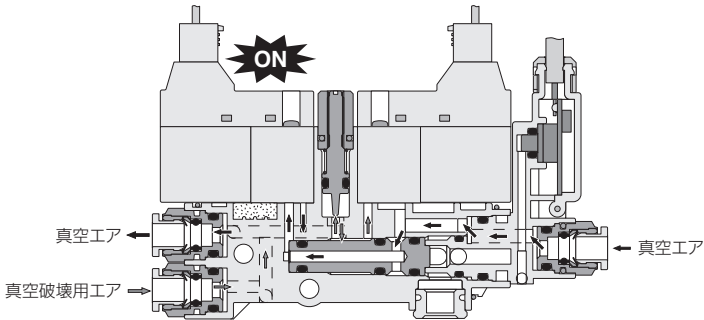
②.真空供給用電磁弁ON時(真空供給状態)
