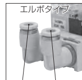
真空破壊用 エア供給ポート 真空供給ポート
