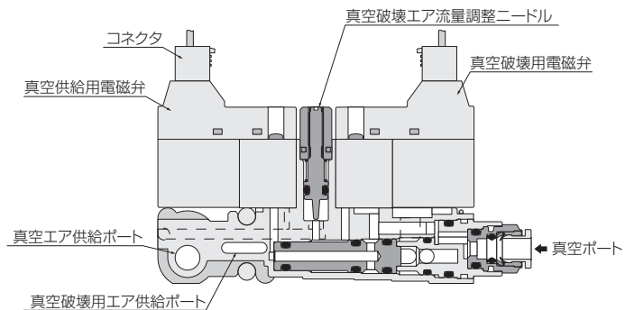
マニホールドタイプ 圧力センサ無し
