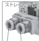
真空破壊用 エア供給ポート 真空供給ポート
